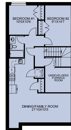
Basement Suite
